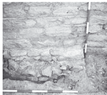
Abb. 46: Raum 34a, Südmauer mit Fundamentgrube SE 1008
